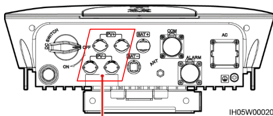
Gleichstromeingangsklemmen
